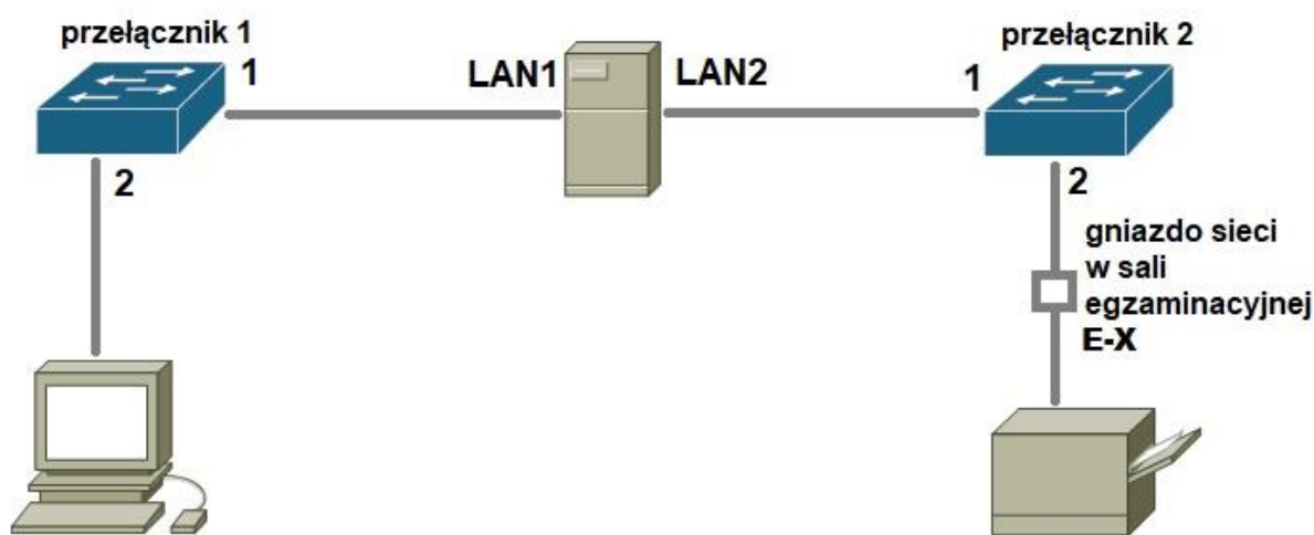
Schemat połączeń urządzeń w sieci lokalnej
