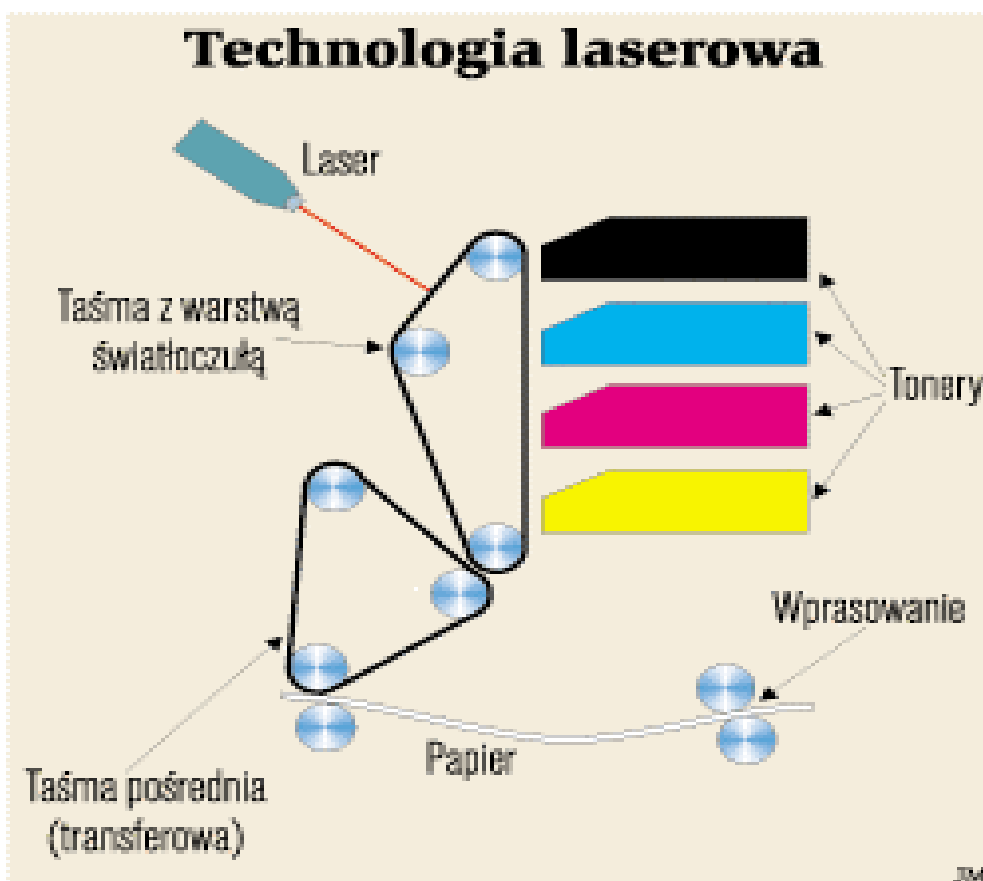
Schemat działania kolorowej drukarki laserowej.
