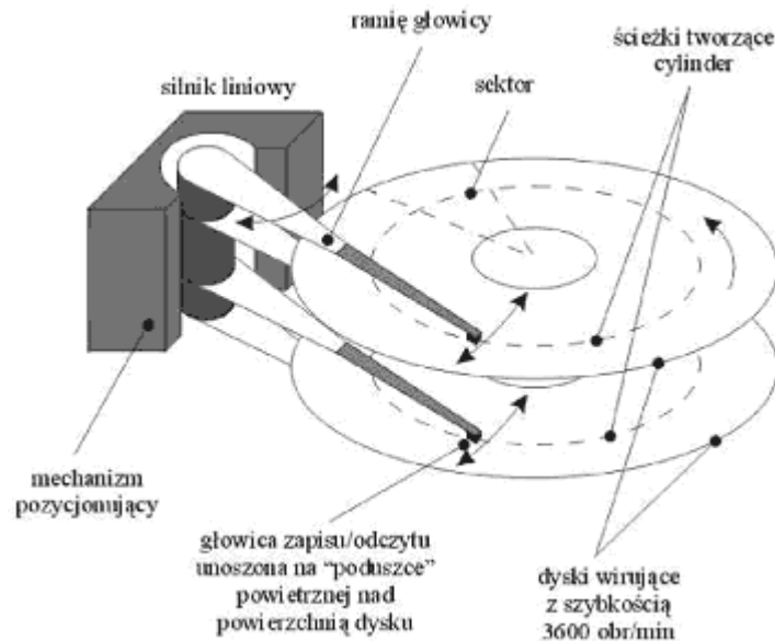
Rysunek 1. Schemat i elementy dysku twardego
